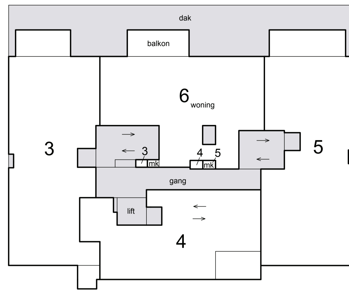
1e etage
